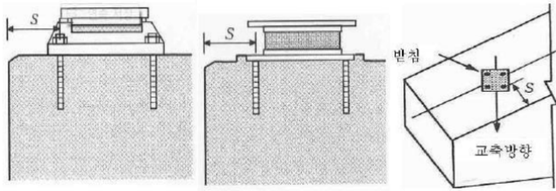
【그림 3.2.17】 교량반침 연단거리
