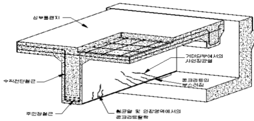
【그림 3.2.5】 철근콘크리트 거더의 조사부위
