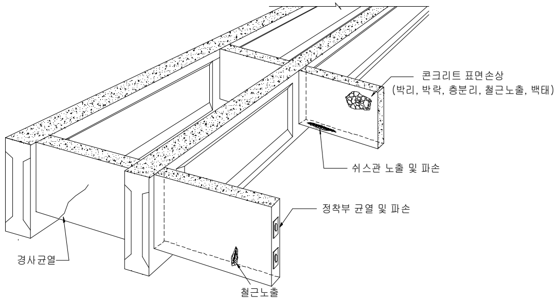
【그림 3.2.7】 콘크리트 가로보 조사부위 및 조사사항
